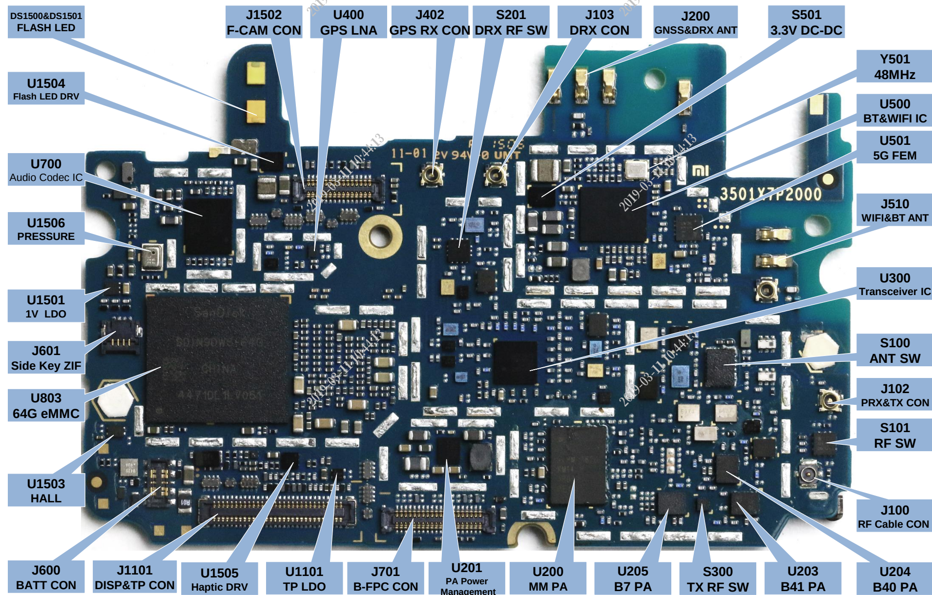
元件分布图-BOTT
