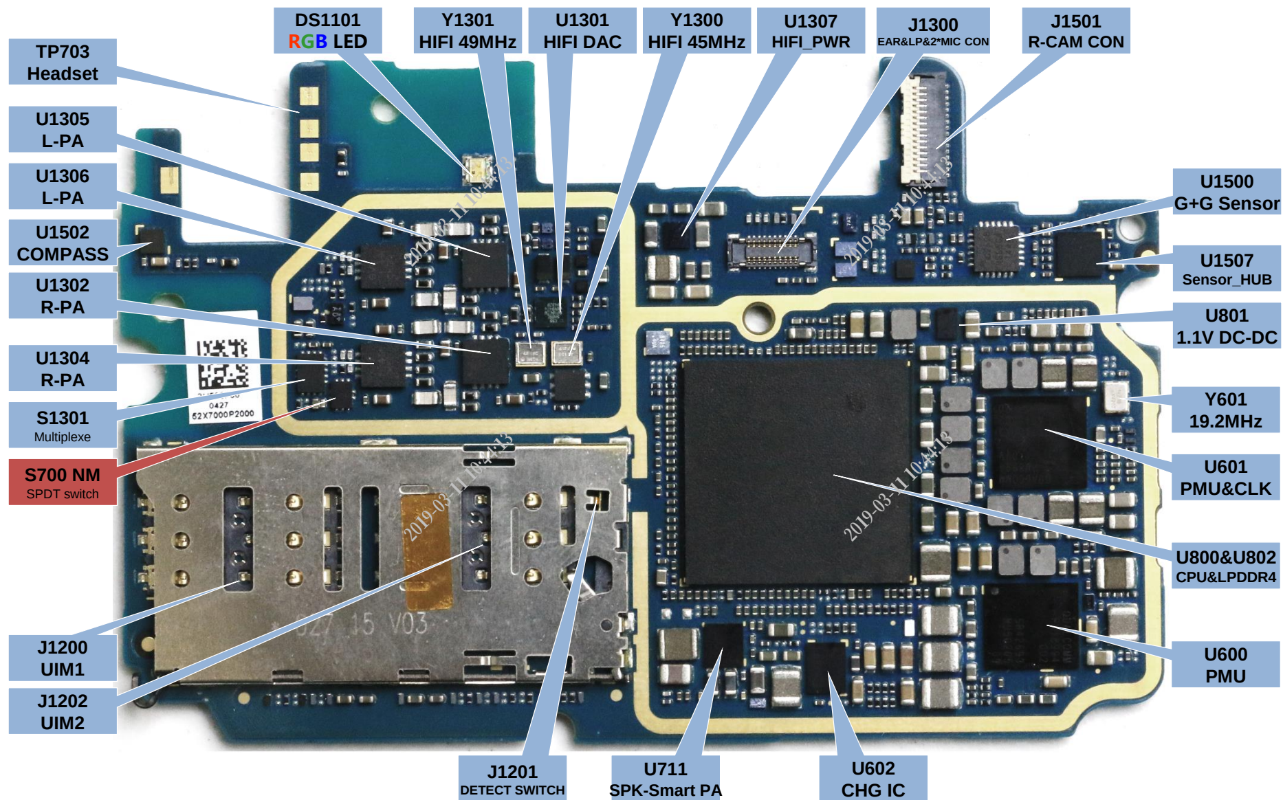
元件分布图-TOP
